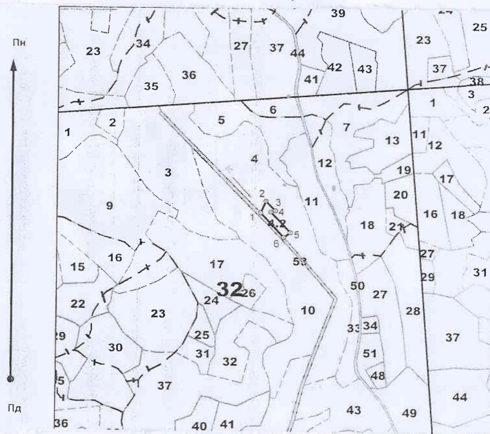
Прив'язка пробних площ (схема)
